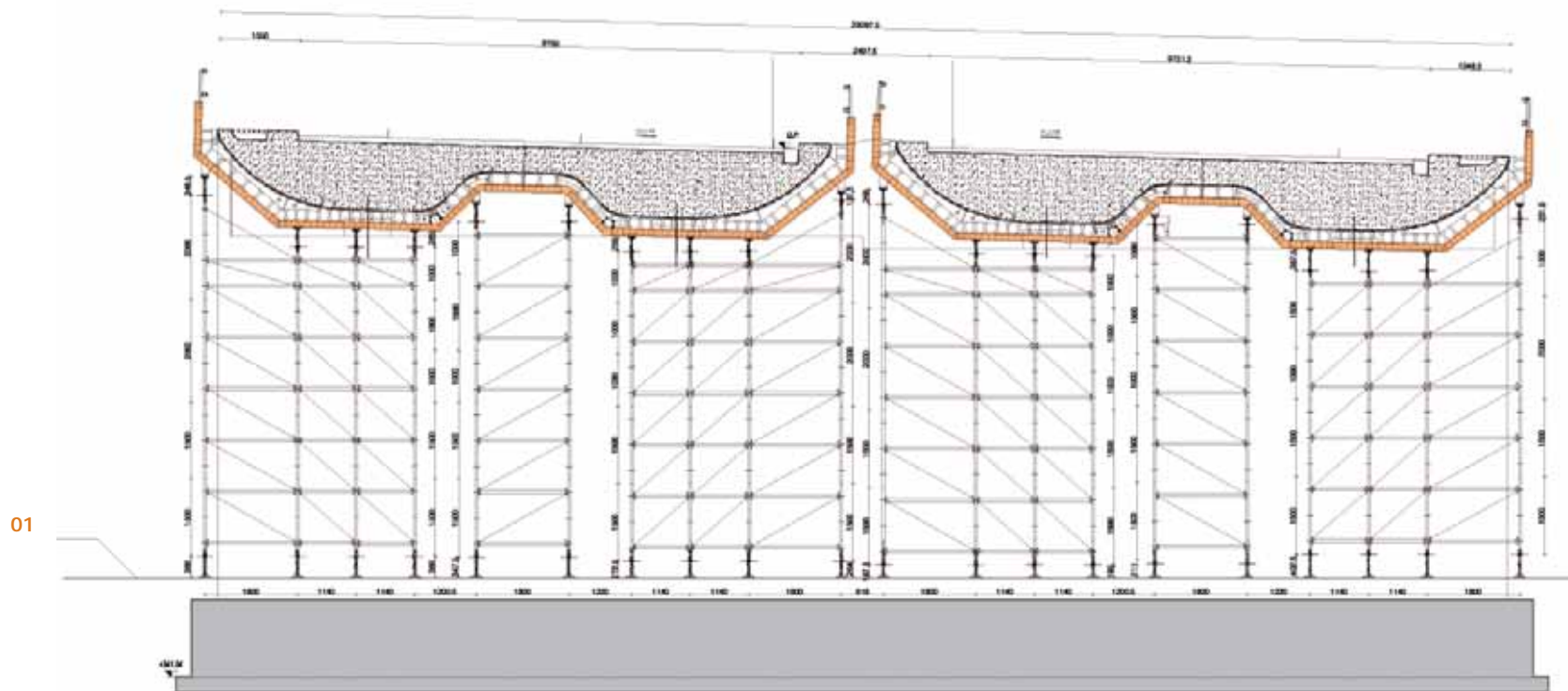
SEZIONE TRASVERSALE - Cross section
